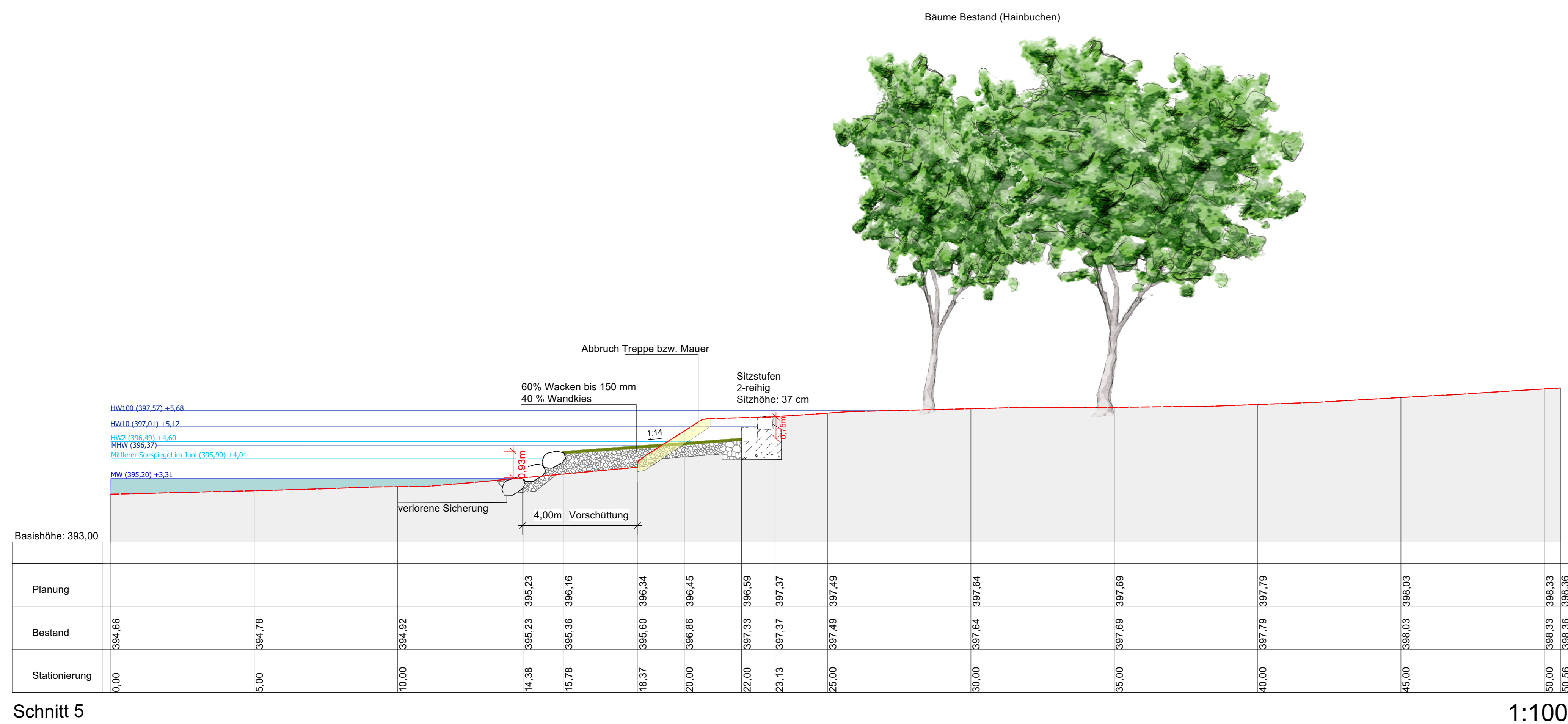
Schnitt 5 1:100
