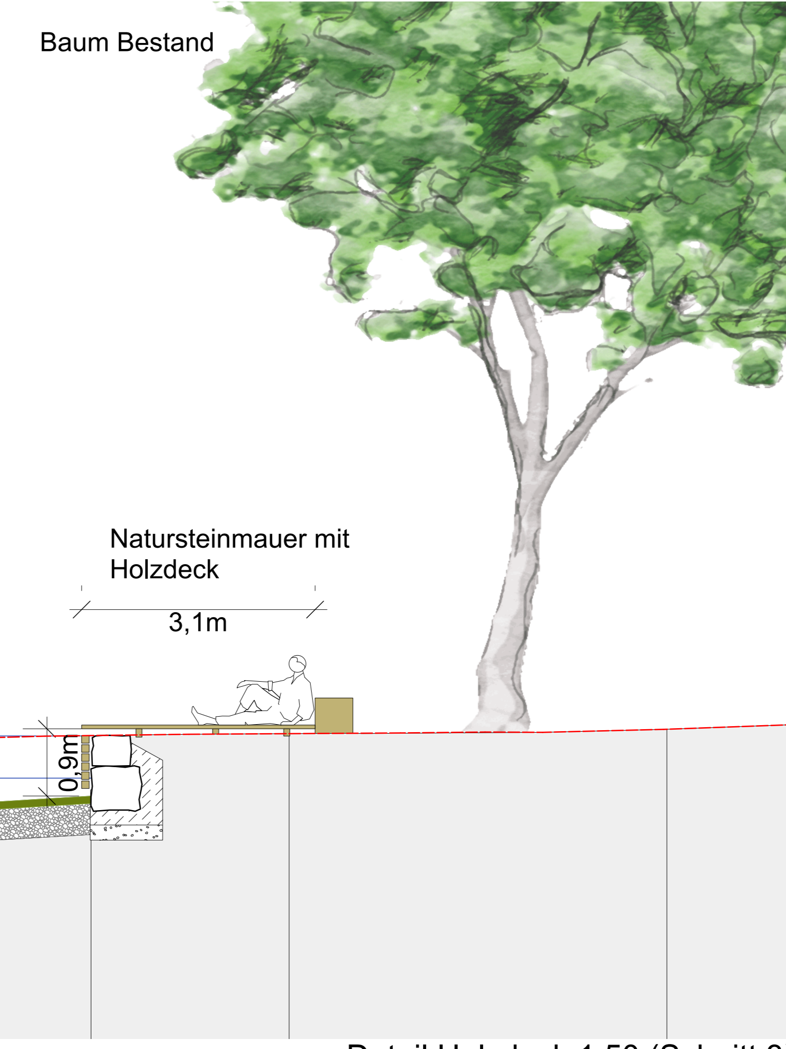
Detail Holzdeck 1:50 (Schnitt 3)
